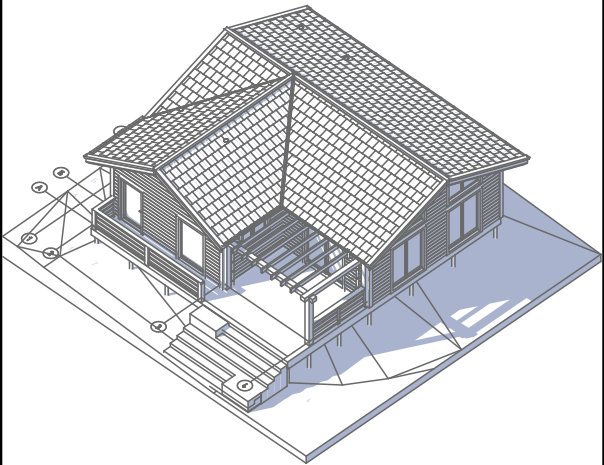
Аксонометрия крыши
