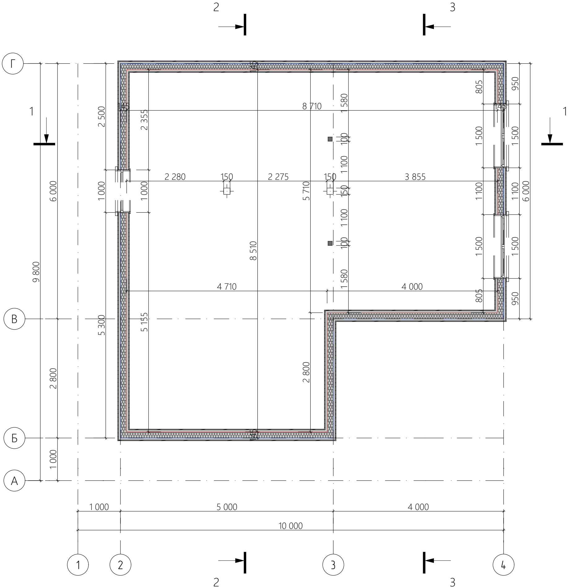
Размерный план 2 этажа
