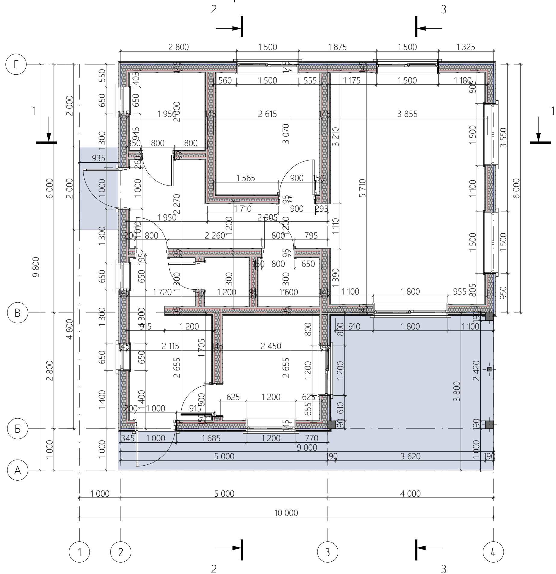
Размерный план 1 этажа
